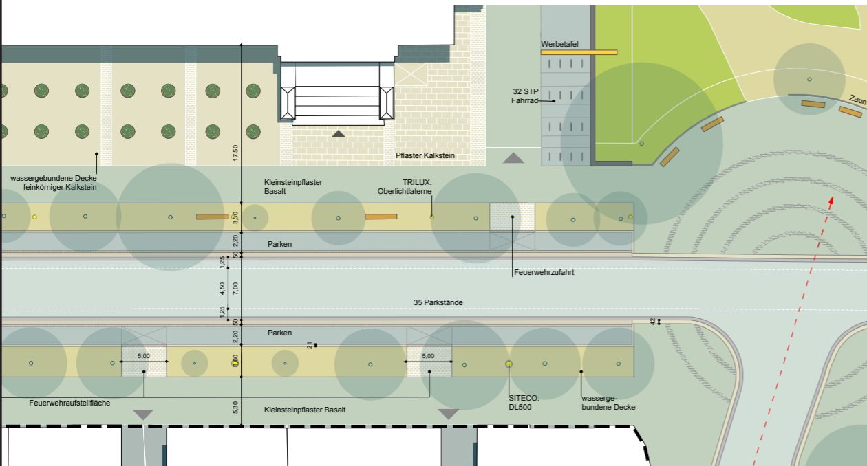
Detailausschnitt
